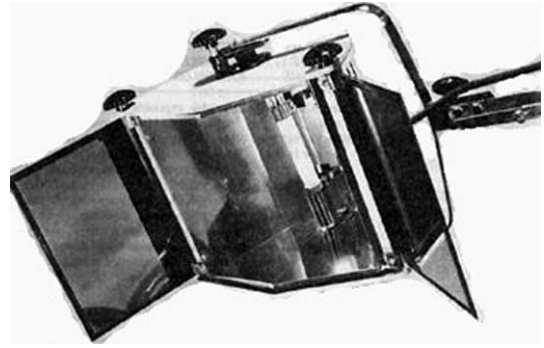
Figura 28.3. Lámpara ultravioleta de “cuarzo caliente” donde se aprecia el quemador y el reflector. Tiene la posibilidad de limitar el área de exposición con las aletas del reflector. Sin embargo la radiación puede escapar.
