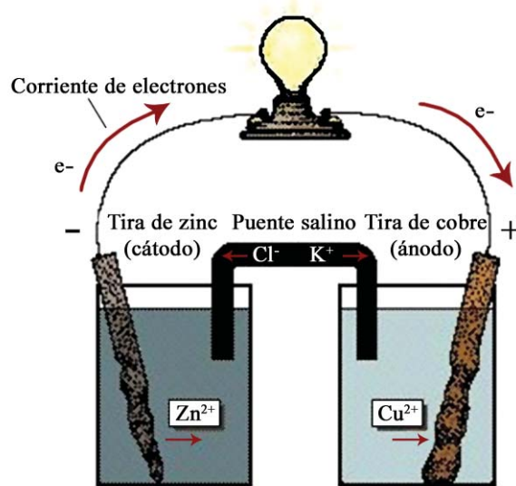
Figura 20. 2. Funcionamiento de una pila electroquímica o pila voltaica. Al colocar una tira de zinc y una tira de cobre en una disolución diluida de ácido sulfúrico, el zinc, que es un reductor, se oxida fácilmente, pierde electrones y los iones zinc positivos se liberan en la disolución, mientras que los electrones libres que quedan en la varilla de zinc, luego pasan al electrodo de metal (cobre) colocado en la disolución. Los electrones que están en este circuito fluirán hacia la disolución, donde serán atrapados por los iones hidrógeno positivos del ácido diluido. La combinación de iones y electrones produce gas hidrógeno, que aparece como burbujas en la superficie del electrodo. La reacción de la varilla de zinc y el ácido sulfúrico produce así una corriente en el circuito externo que se puede percibir en la bombilla.
