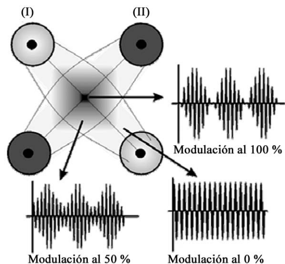
Figura 23.1. Corrientes de media frecuencia. En la zona donde se produce el cruce de los circuitos se obtiene una corriente modulada cuya frecuencia oscila entre 0 y 200 Hz, equivalente a la diferencia de las frecuencias de las dos corrientes iniciales; sus efectos excitomotores son semejantes a los producidos por las corrientes de baja frecuencia. Esta corriente se denominó corriente interferencial; su intensidad, al contrario de las corrientes individuales aplicadas, varía rítmicamente.
