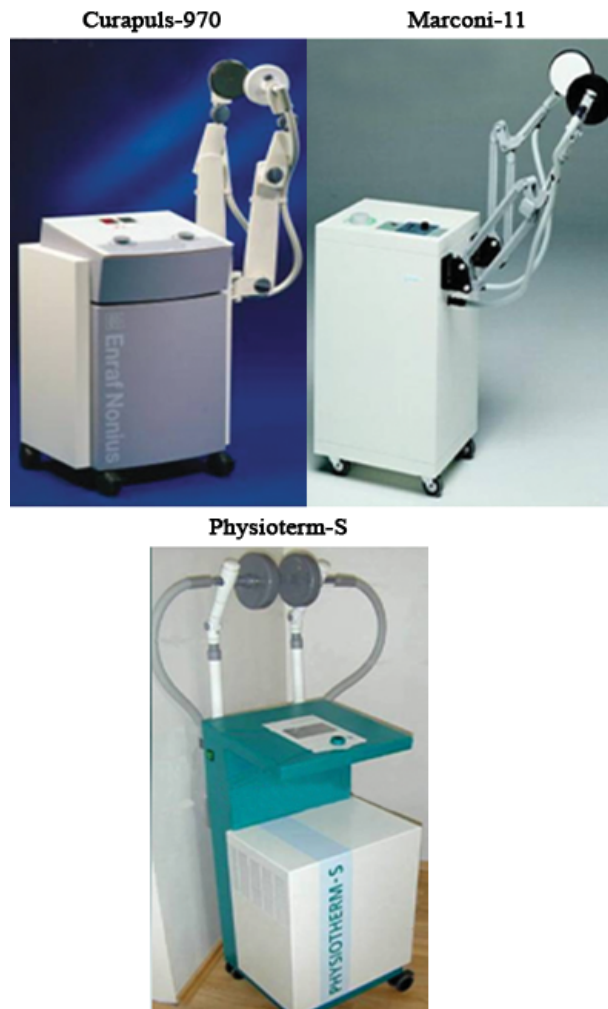
Figura 25.2. Equipos de diatermia por onda corta. Todos estos equipos de electroterapia de alta frecuencia, cuentan con brazos para ayudar en la ubicación de los aplicadores en la zona corporal a tratar.
