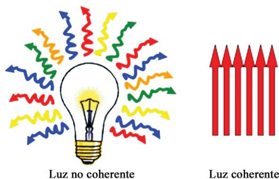
Figura 30.3. Esquema que muestra la diferencia entre un bombillo incandescente convencional (izquierda) y una emisión del haz láser (derecha). El bombillo emite radiación de muchas longitudes de onda. Solo los fotones que emite dentro de la región visible del espectro, tienen un color específico. Cada fotón se va a desplazar en diferentes fases. La resultante es una luz de color predominantemente amarillo. De manera que el bombillo emite una luz no polarizada o no coherente.
