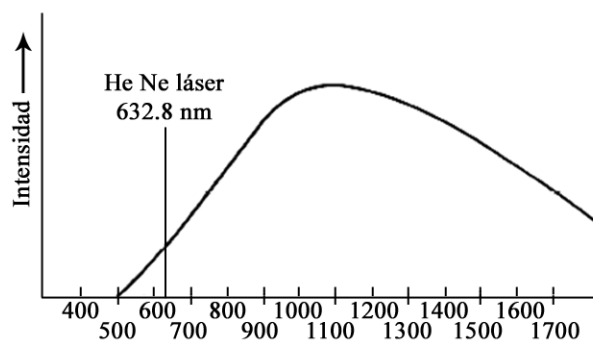
Figura 30.4. Esquema que muestra una comparación entre la salida de un láser He-Ne y una lámpara infrarroja.
