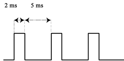
Figura 22.1 Esquema de la corriente de Träbert. Se trata de una corriente monofásica con impulso cuadrangular.
